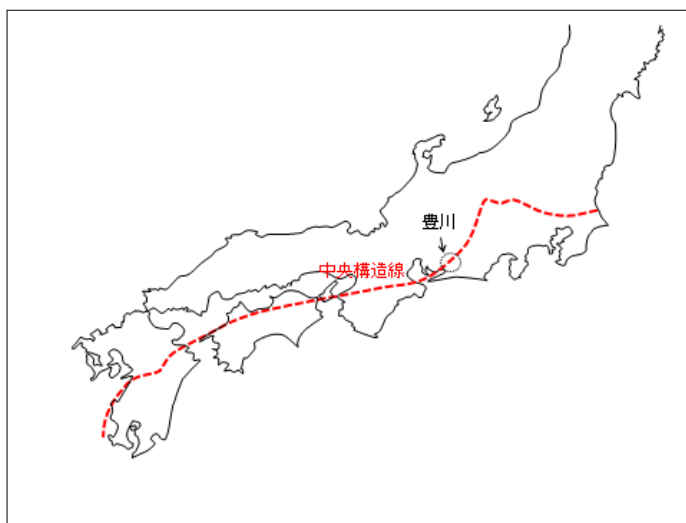
図. 3 中央構造線の略図
