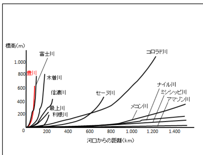
図. 4 河川の勾配
